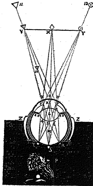
Abb. 1 Der Strahlengang im Linsenauge (nach Descartes, Dioptrique )
